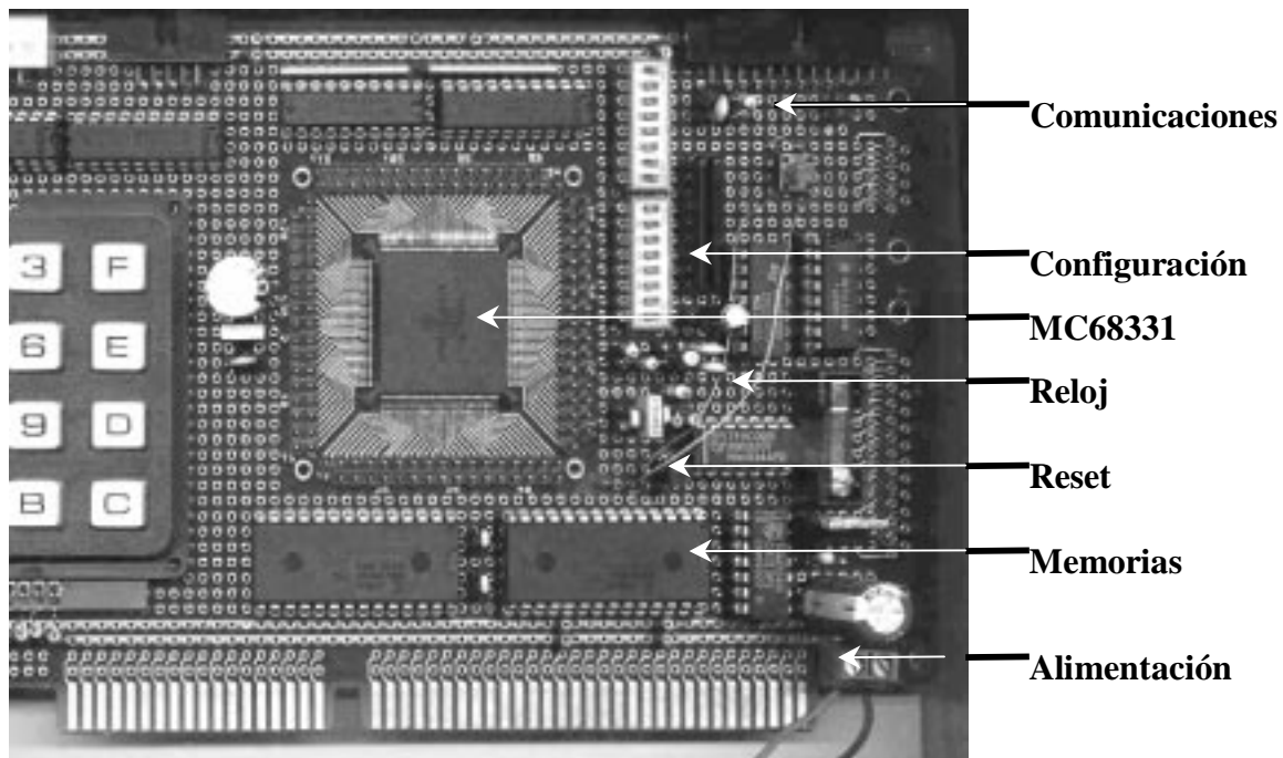
Figura 1: Detalle de una de las tarjetas construidas por los alumnos
